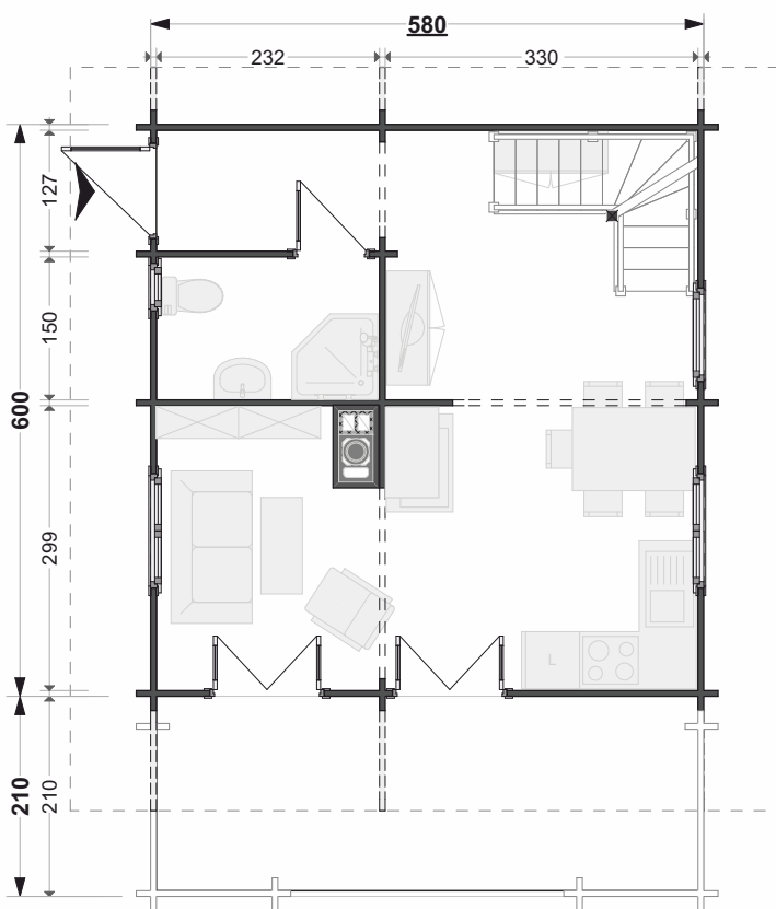
Prízemie / Ground floor
