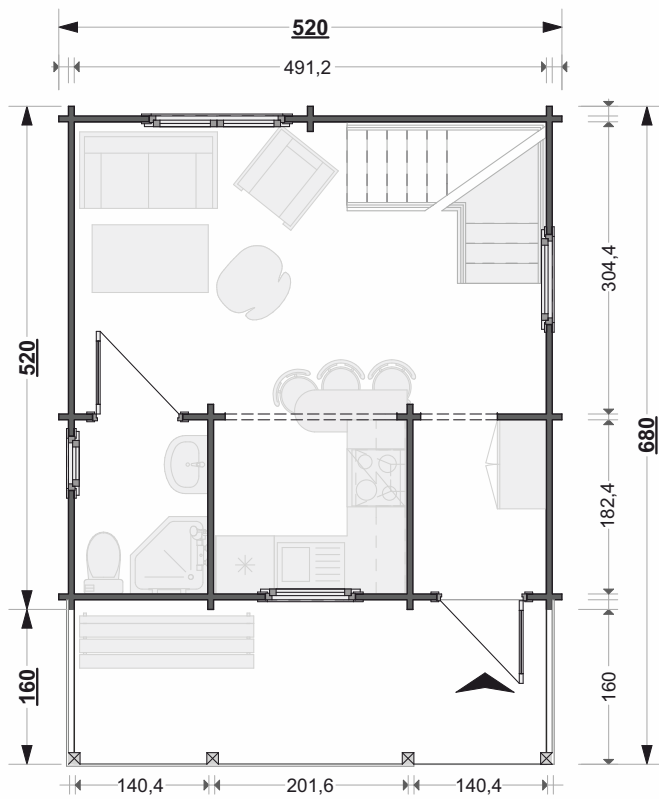
Prízemie / Ground floor
